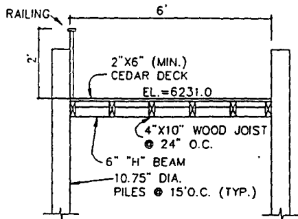
WALKWAY SECTION N.T.S.
