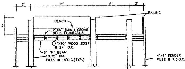
PIERHEAD SECTION N.T.S.
